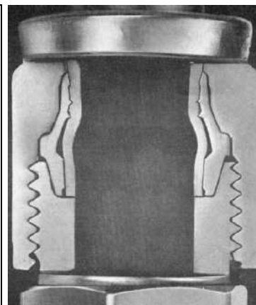
Conexión Sello Perfecto después de repetidos ensambles. Nótese cómo el segundo "diente" sujeta ahora al tubo. El sello perfecto se mantiene aun después de repetido ensambles sin afectar al tubo.
